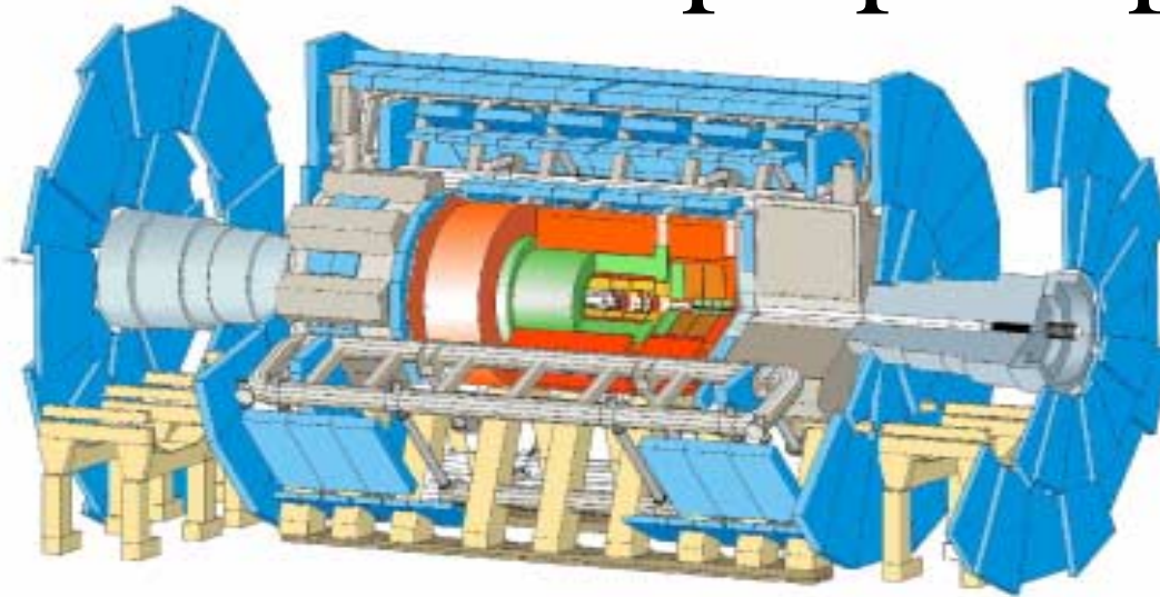
ATLAS
